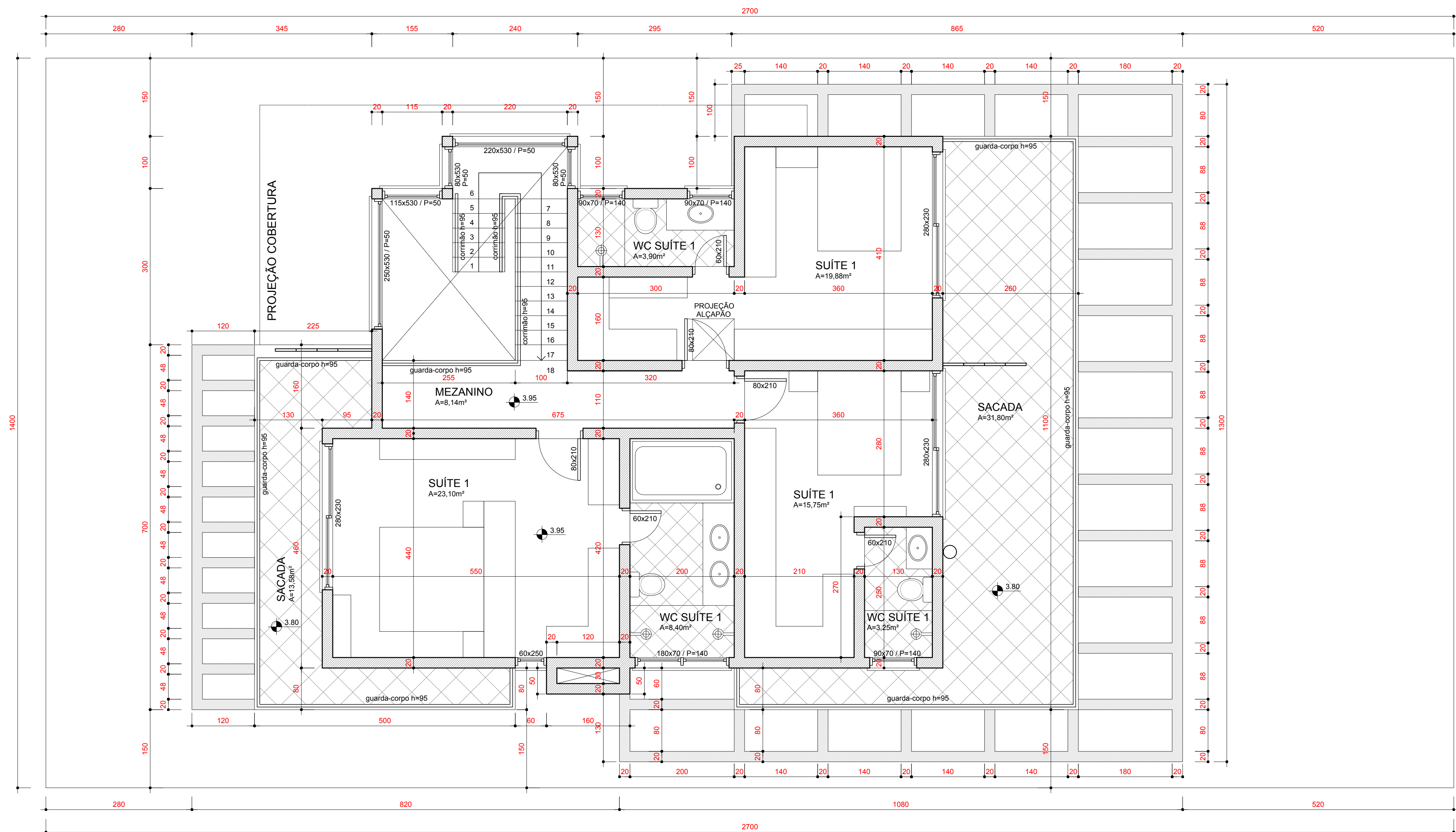
PLANTA BAIXA 2º PAV. ESCALA 1/50 A=96,74m² A total =251,03m²
