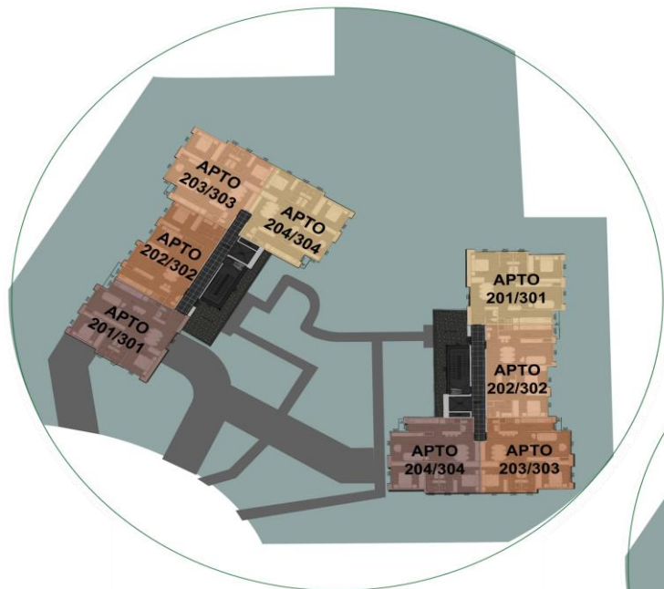
PLANTA BAIXA TIPO
