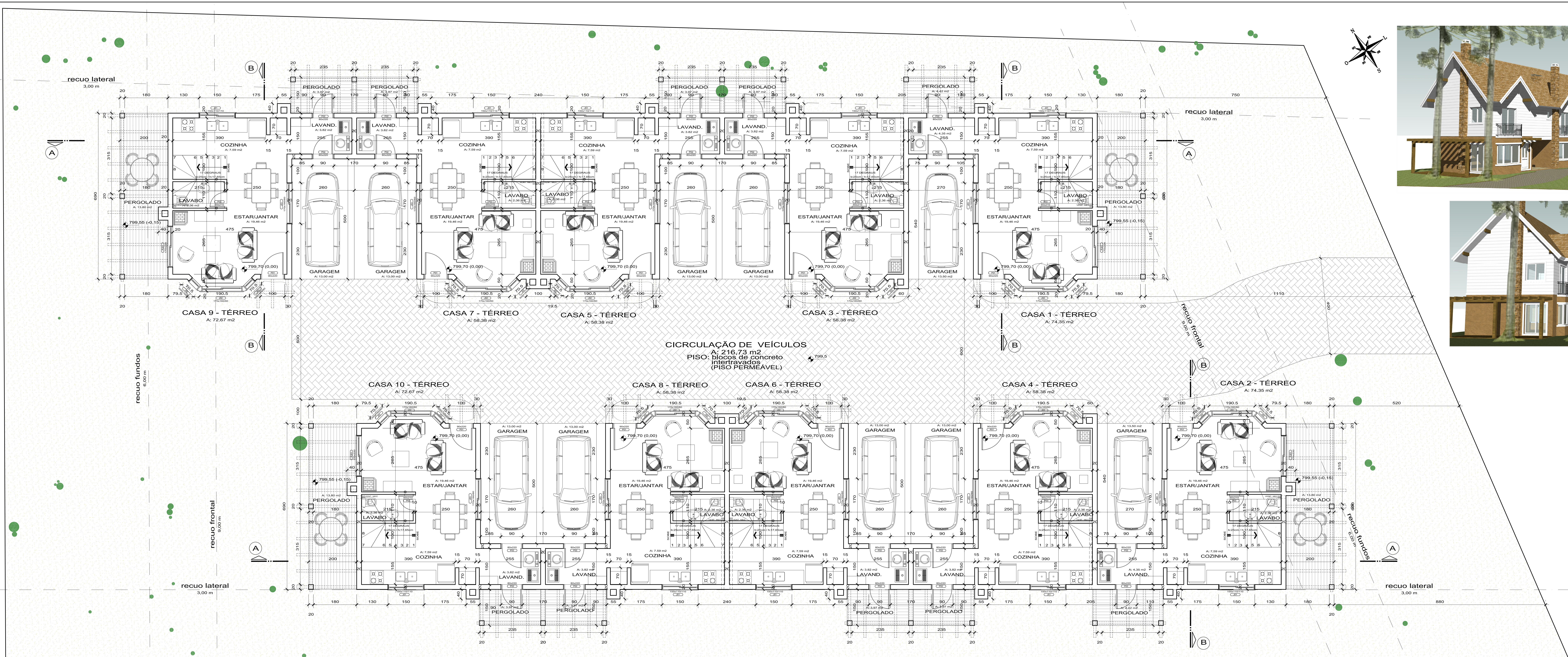
PAV. TÉRREO ESC.: 1:50
