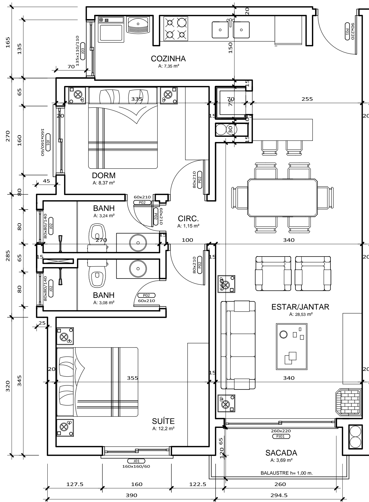
TORRE SOLARIS - APARTAMENTO 105-205 ÁREA: 74,63m 2
