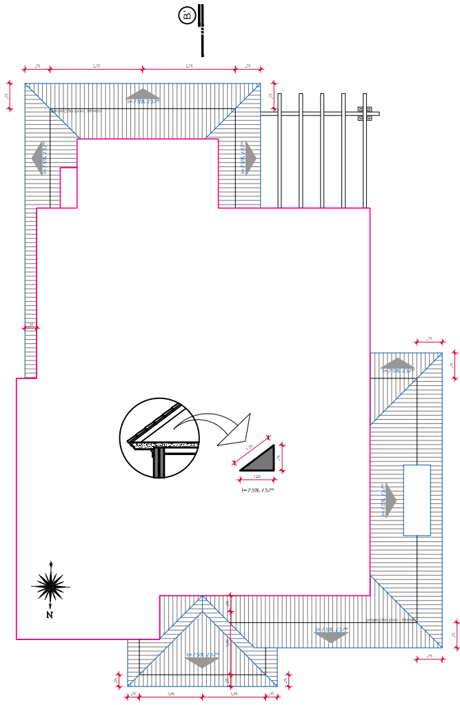
PLANTA COBERTURA PAV. TÉRREO
