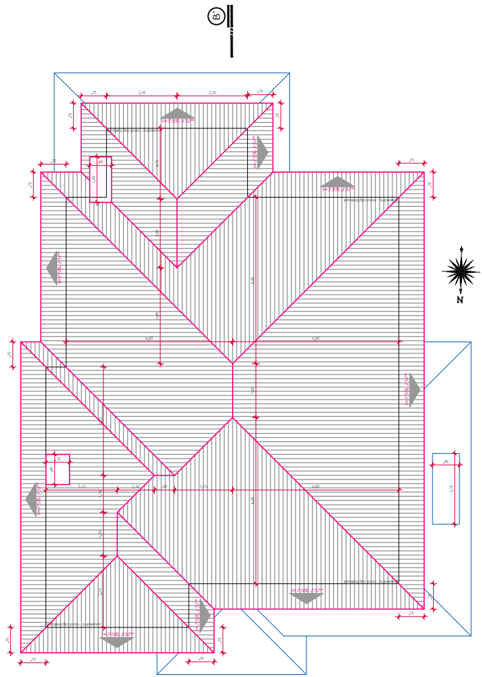
PLANTA COBERTURA PAV. SUPERIOR
