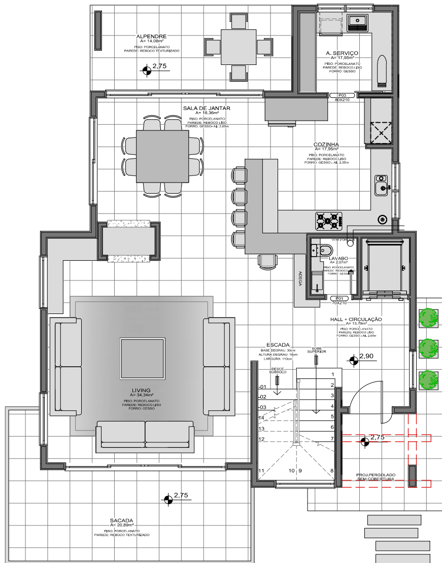
PAVIMENTO TÉRREO A = 138,45m 2
