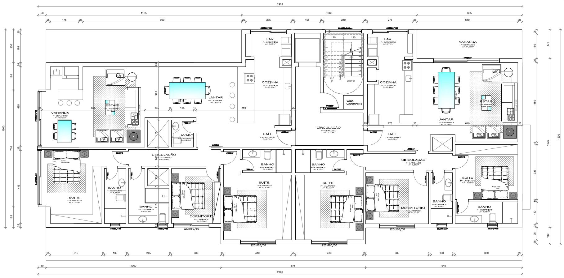
PL. COBERTURA A= 249,09m 2 Esc.: 1/75
