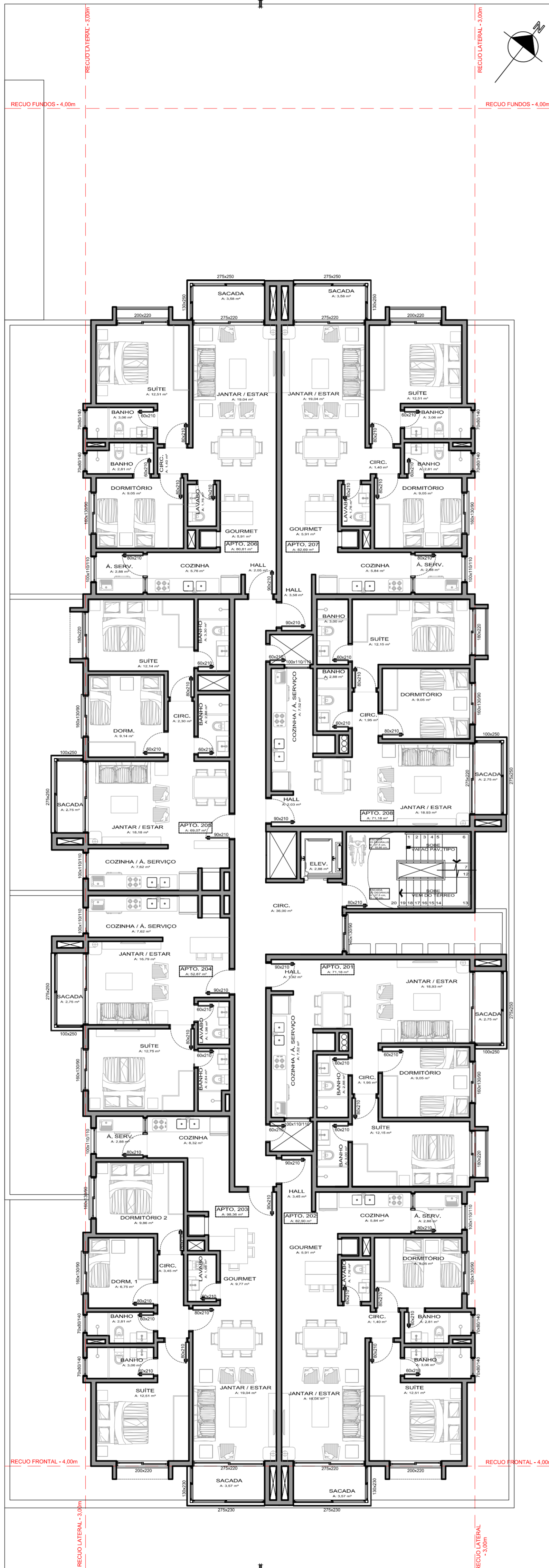
PLANTA BAIXA 1º PAVIMENTO Área : 686,79m² ESCALA 1/100
