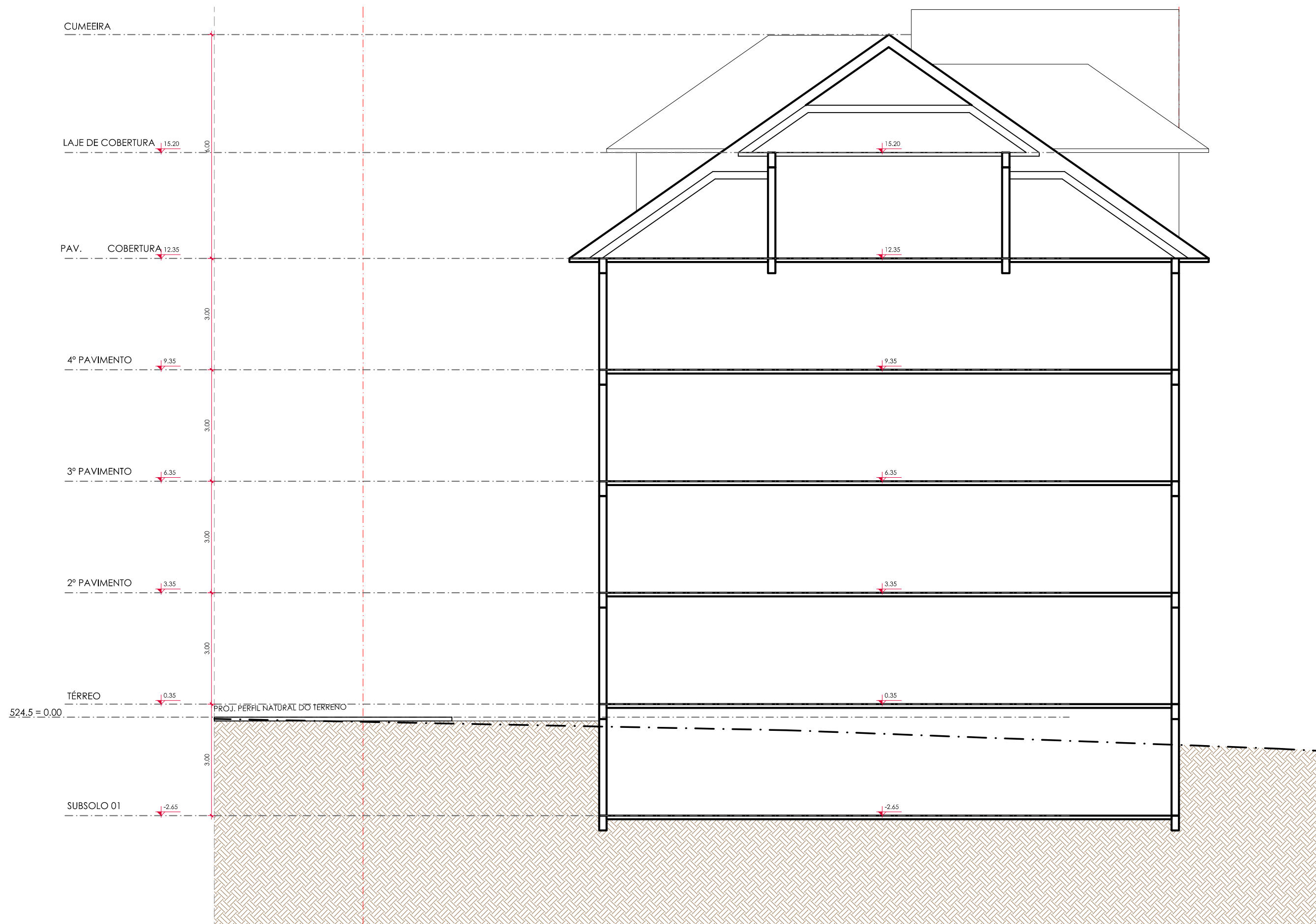
CORTE BB SCALA: 1/100
