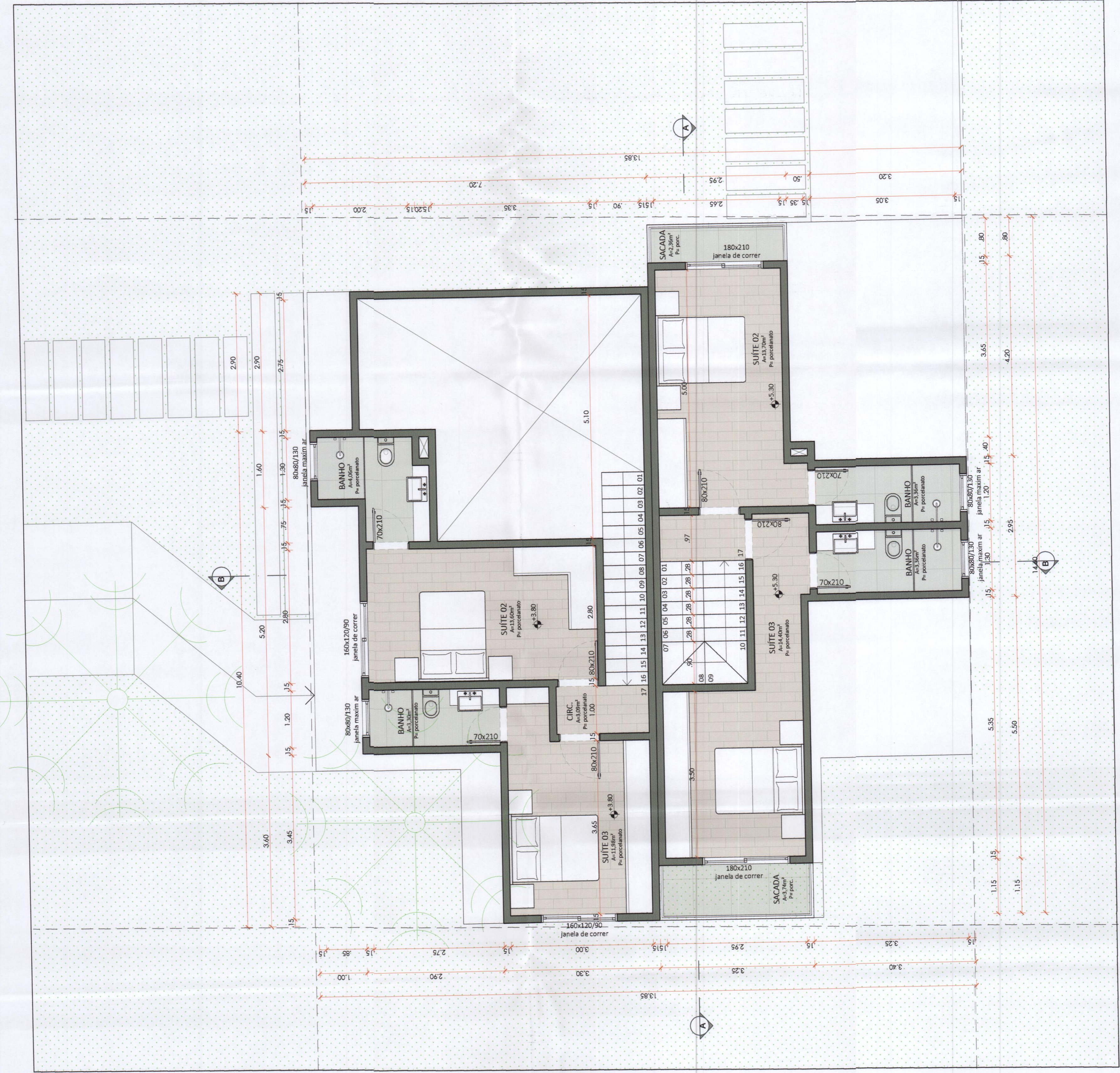
Planta baixa segundo pavimento Escala 1/50
