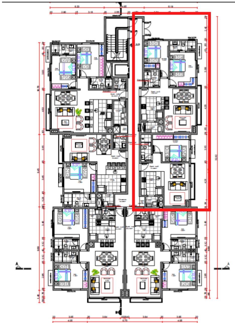
Bloco 1 (Torre Pisa) - Térreo
