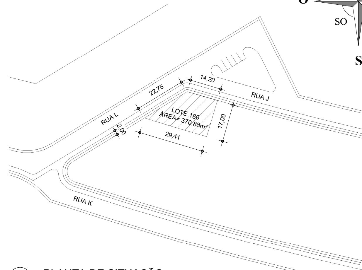
2 PLANTA DE SITUAÇÃO ESCALA 1 : 1000
