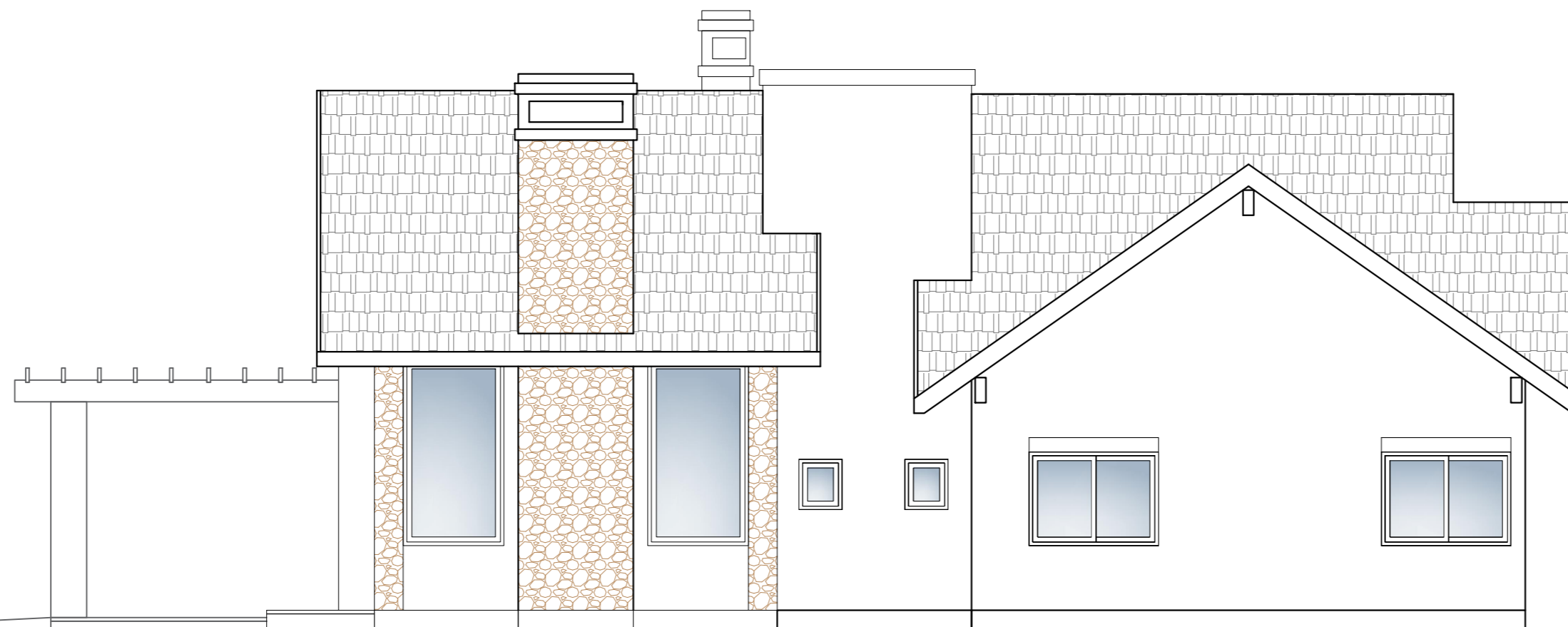
FACHADA LATERAL DIREITA ESCALA: 1/75
